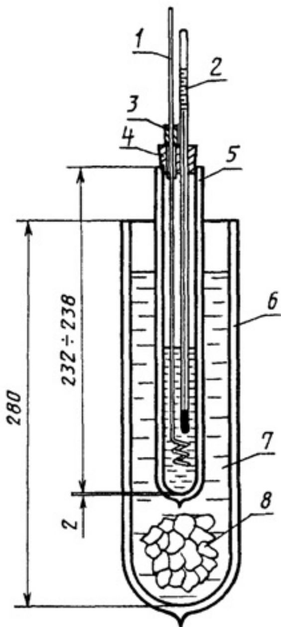
1 - мешалка; 2 - термометр; 3 - уплотнение; 4 - пробка; 5 - сосуд для пробы; 6 - сосуд для измерения помутнения; 7 - сосуд для мешалки; 8 - сетчатый фильтр для мешалки.
