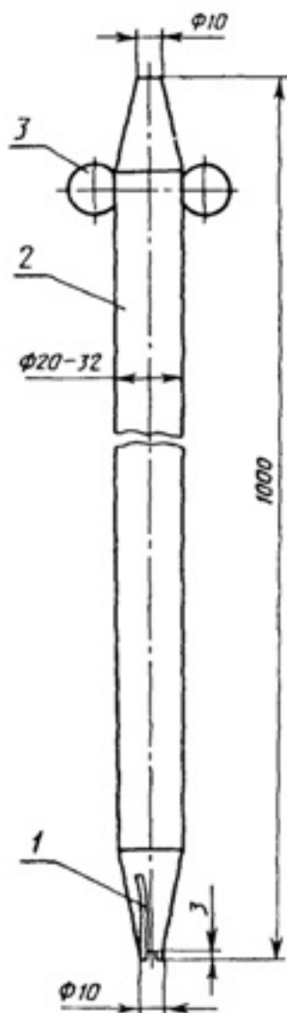
Вид 1 - конус, 2 - трубка, 3 - ушко
