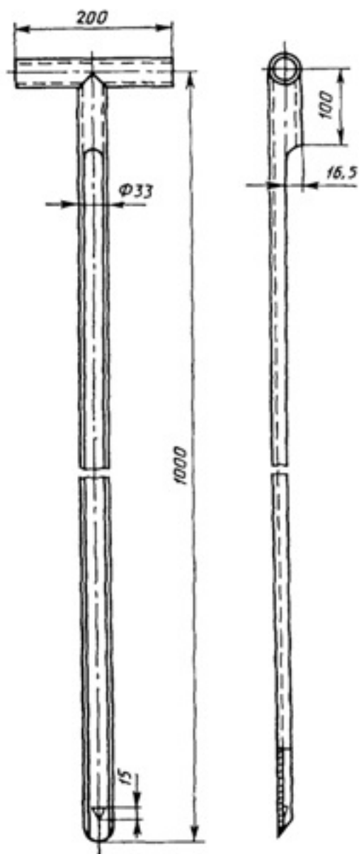
Першневый шуп
