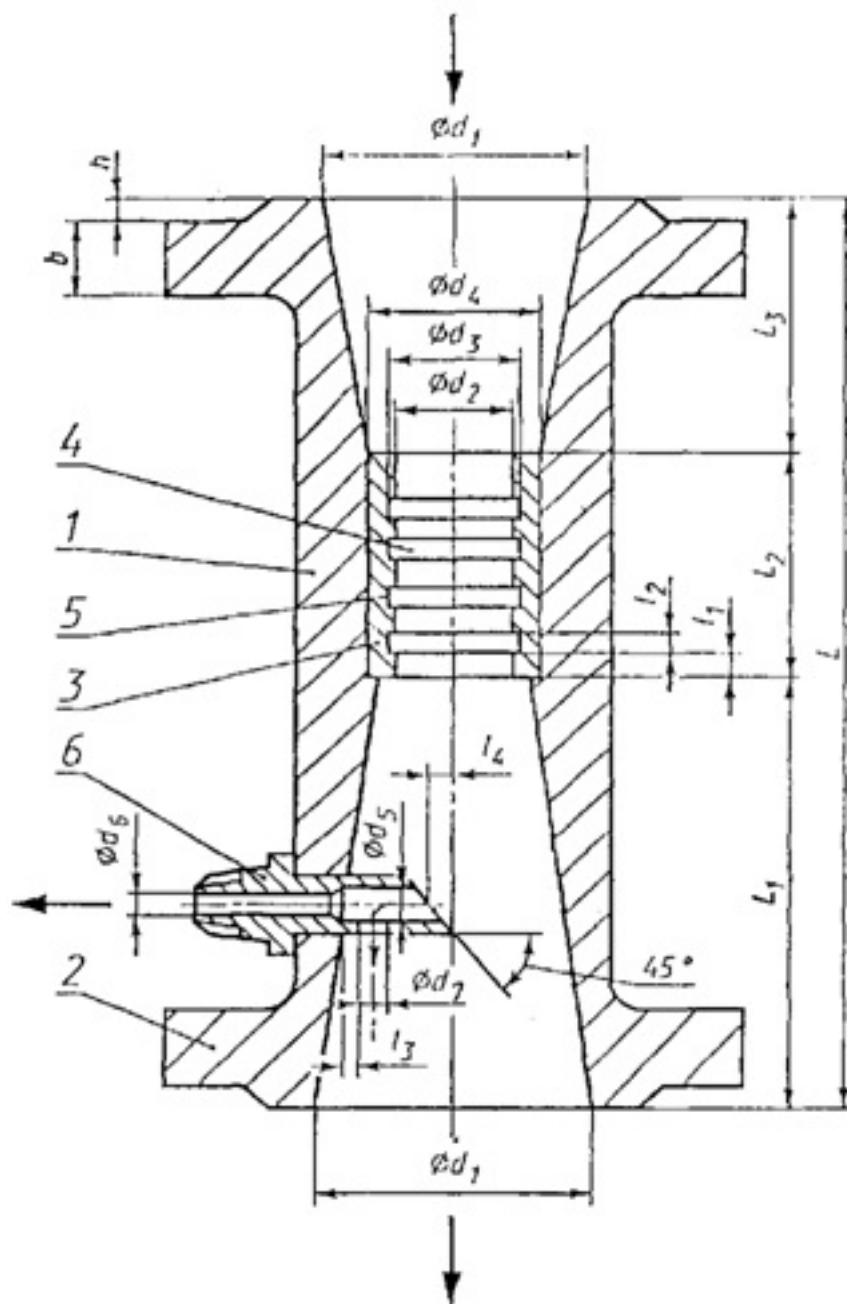
1 корпус; 2 фланец; 3 уплотняющая втулка; 4 и 5 соответствующие отверстия; 6 пробник (численные значения диаметров и длин указаны в приложении 3)
