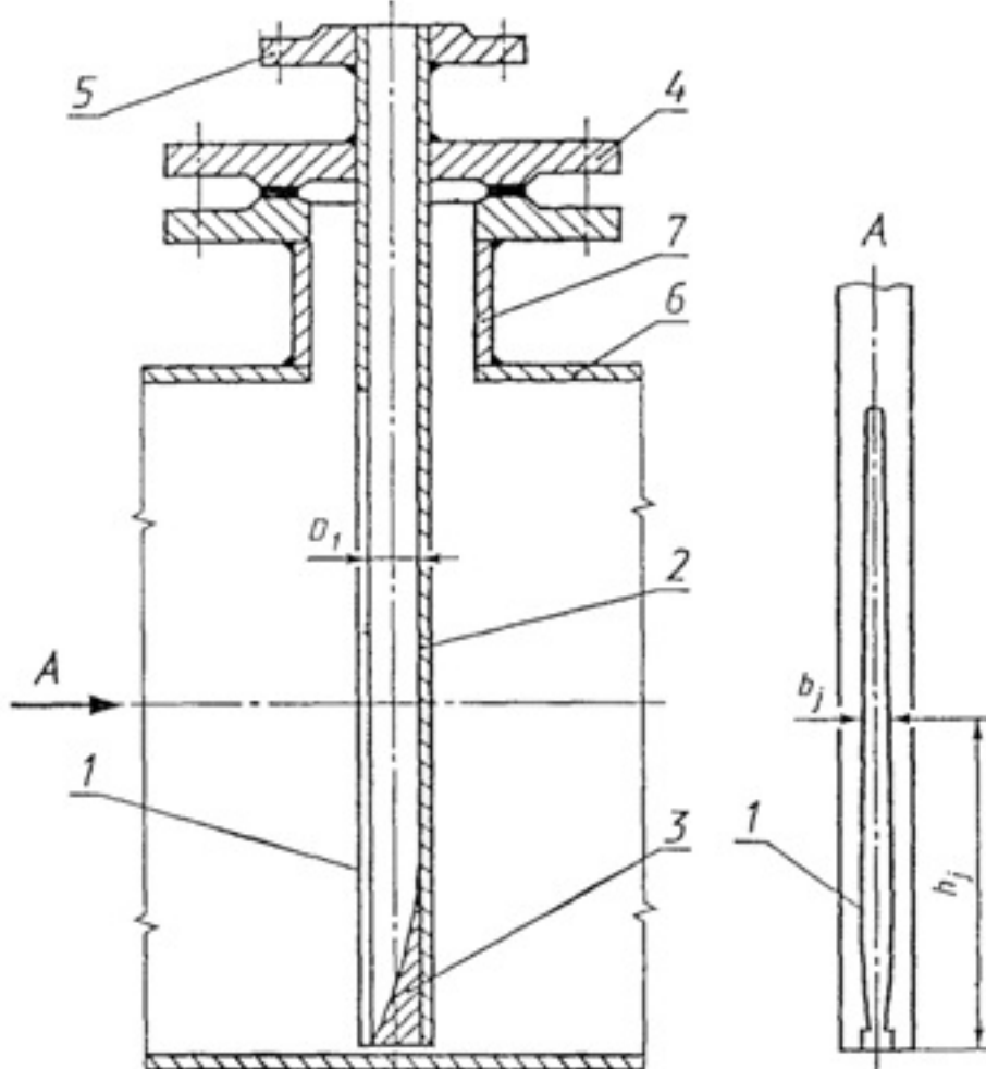
1 - отверстие; 2 - трубка; 3 - стабилизатор; 4 - крышка; 5 - штуцер; 6 - трубопровод; 7 - предохранительный щелевой тип с плавью отверстиями
