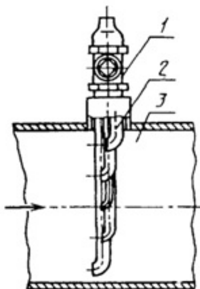
Рис. 1. Схема отбора проб из скважины с помощью зонда
