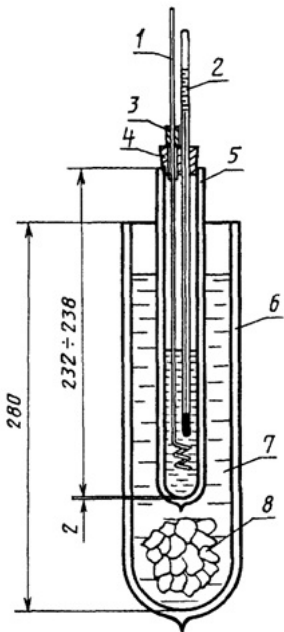
1 - мешалка; 2 - термометр; 3 - уплотнение; 4 - пробка; 5 - сосуд для пробы; 6 - сосуд для измерения помутнения; 7 - сетка; 8 - гранулы для мешалки
