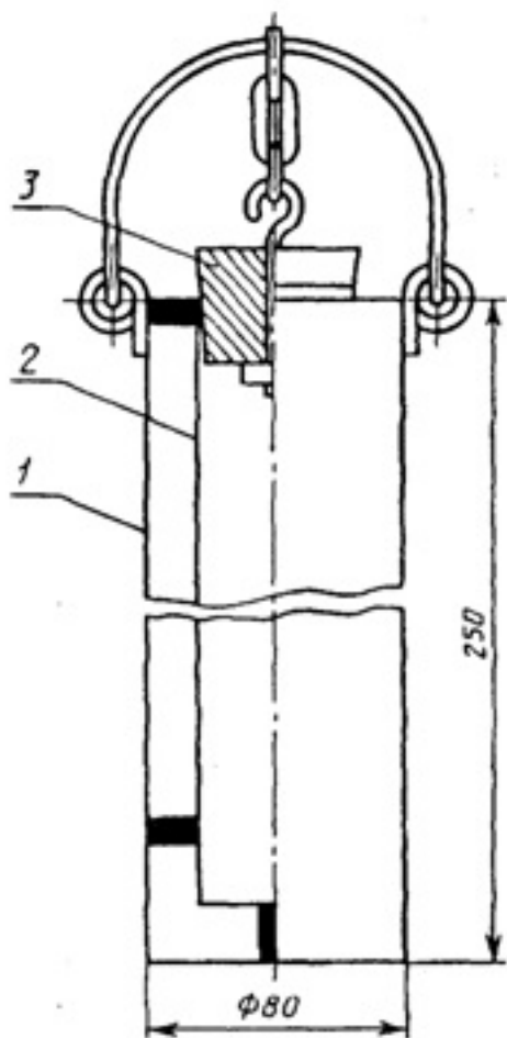
Пробоберная трубка: 2 - внутренний цилиндр; 3 - пробка
