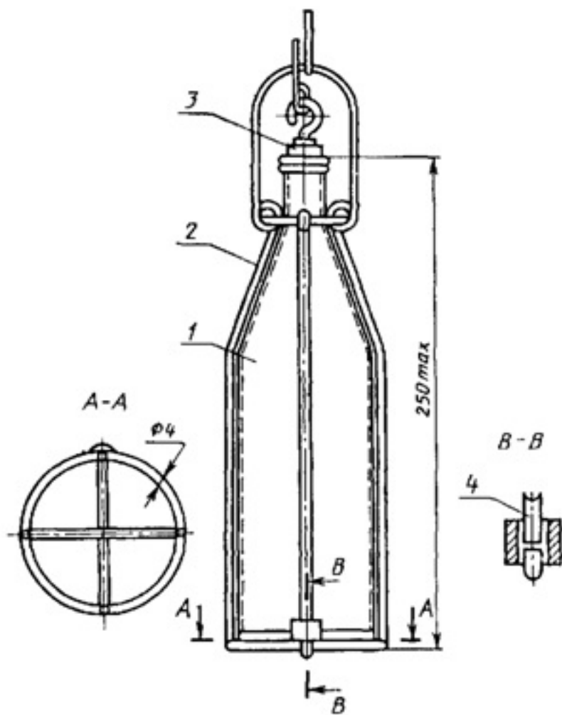
1 - бутылка; 2 - металлический каркас; 3 - пробка; 4 - замок Периодический пробоборник
