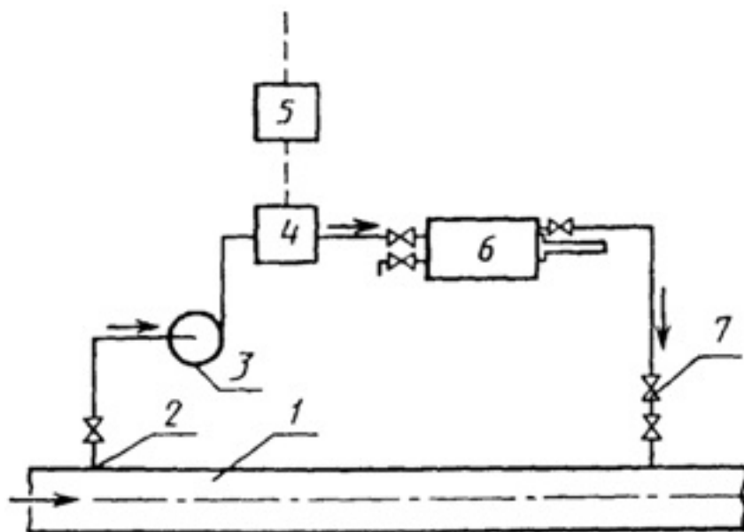
1 - трубопровод; 2 - пробозаборное устройство; 3 - насос; 4 - запорное устройство; 5 - приемная емкость; 6 - фильтр; 7 - обратное устройство
