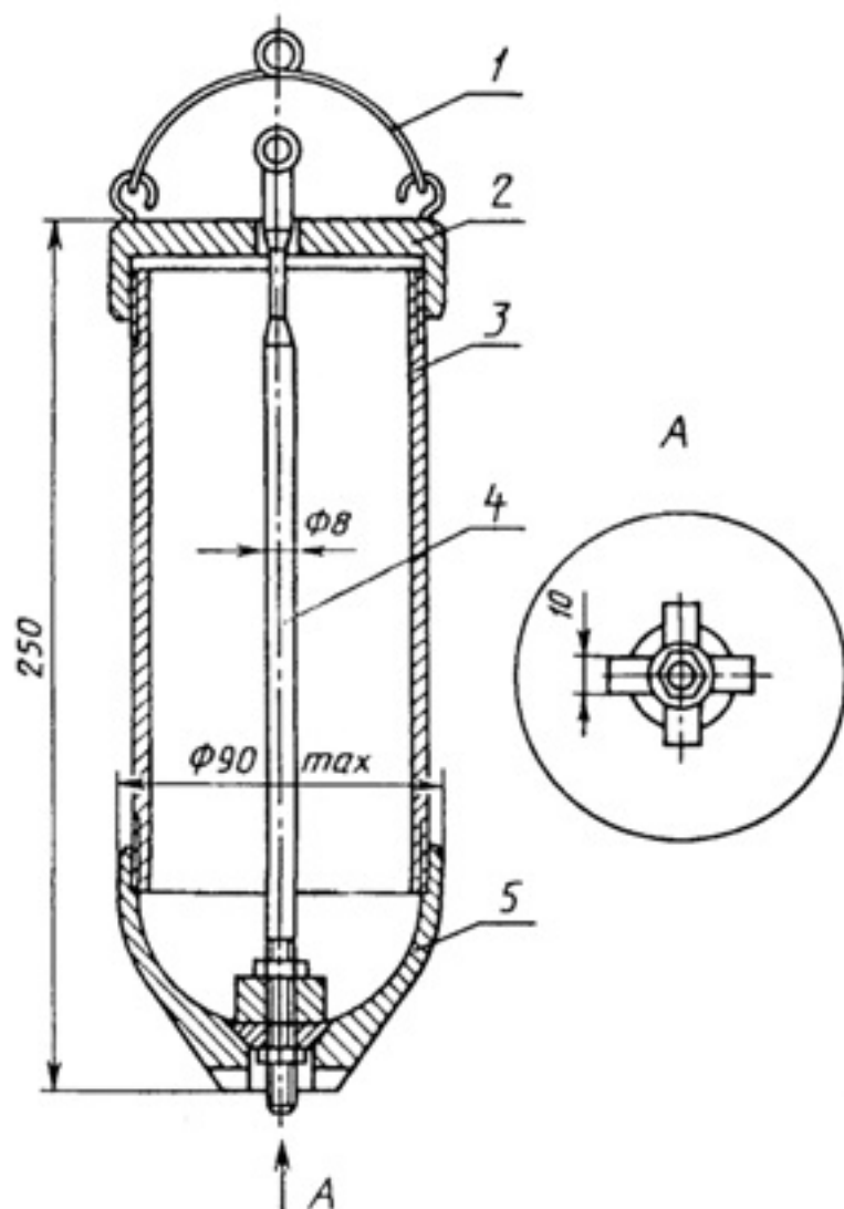
1 - скоба; 2 - крышка с клапаном; 3 - корпус; 4 - шток с клапаном; 5 - днище Бурьяка в металлическом каркасе
