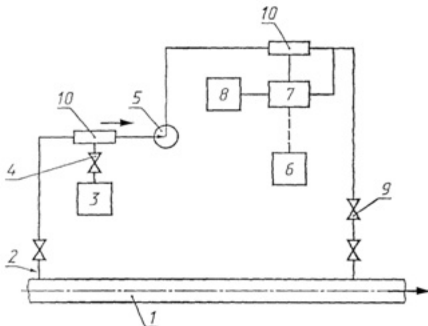
1 - трубопровод; 2 - пробозаборное устройство; 3, 8 - пробозаборники; 4 - кран для отбора проб нефти и нефтепродуктов из трубопроводов; 5 - насос; 6 - фильтр; 7 - запорное устройство; 9 - обратное устройство; 10 - фильтр
