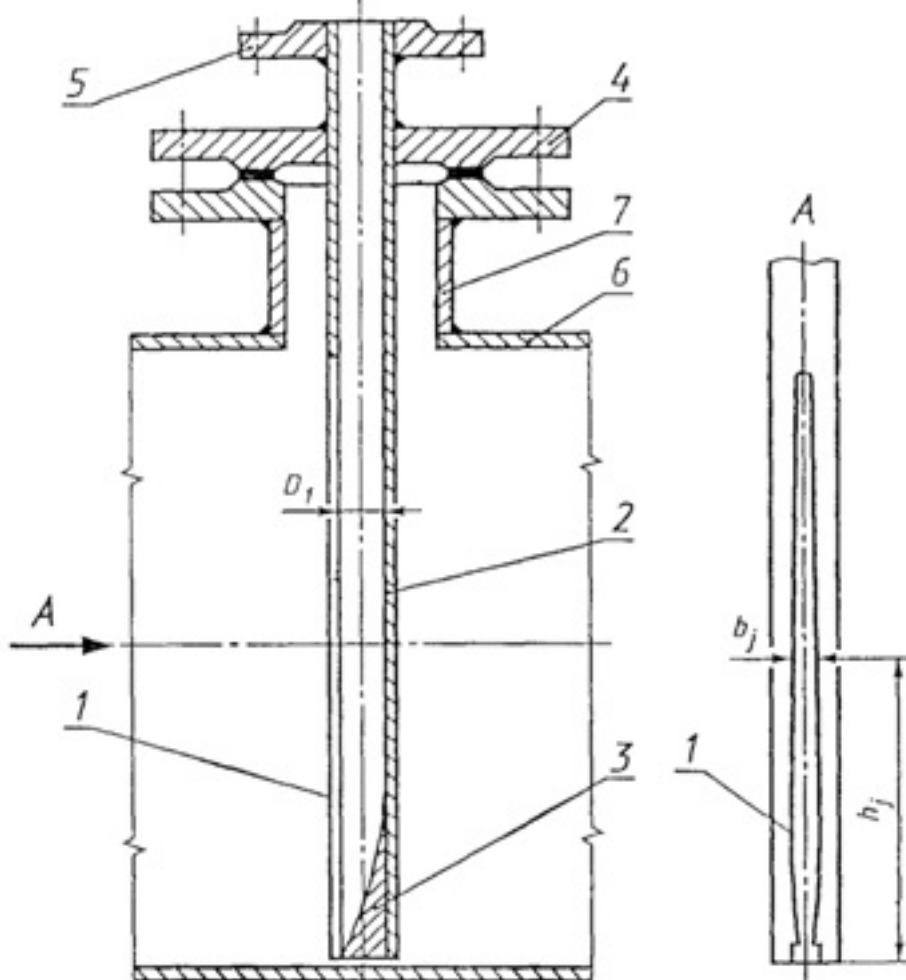
Рис. 1.1.2. Схема отбора проб из скважины с помощью зонда с плавным отверстием
