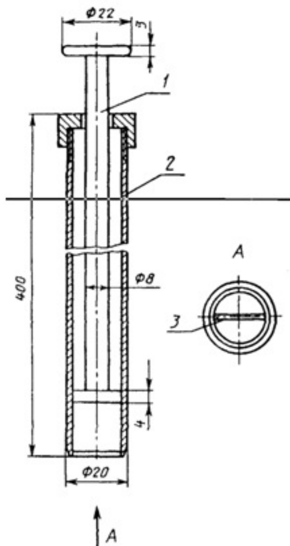
Черт. 1. Прямой без выреза. 2 - корпус из тонкостенной трубки; 3 - проволока
