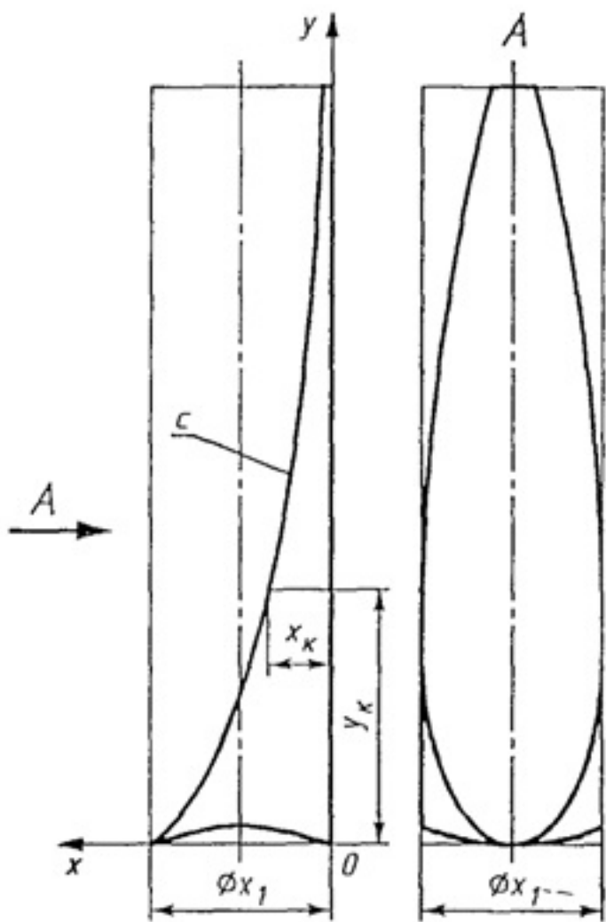
Черт. 20. Изм. 1. Параметры и размеры стабилизатора определяются по алгоритму, приведенному в приложении 2.
